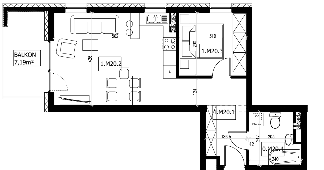
ZESTAWIENIE POMIESZCZEŃ MIESZKANIE- M20
